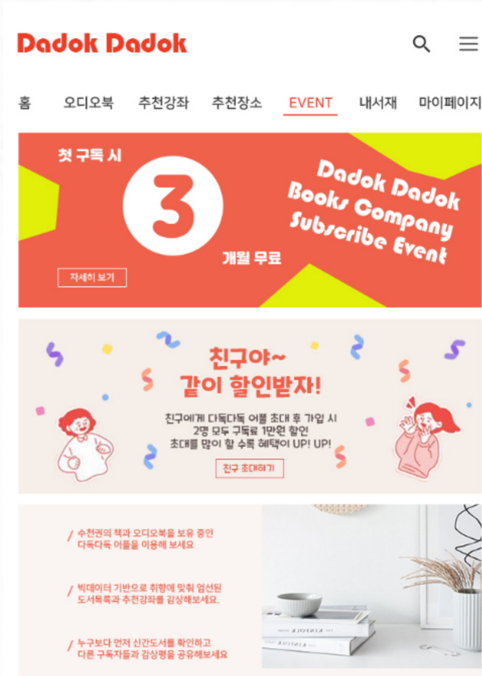
이벤트 상단
