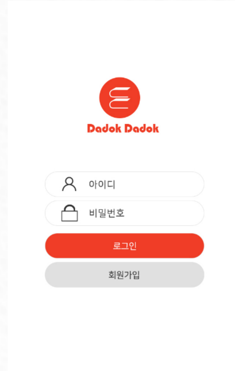
로그인 화면
