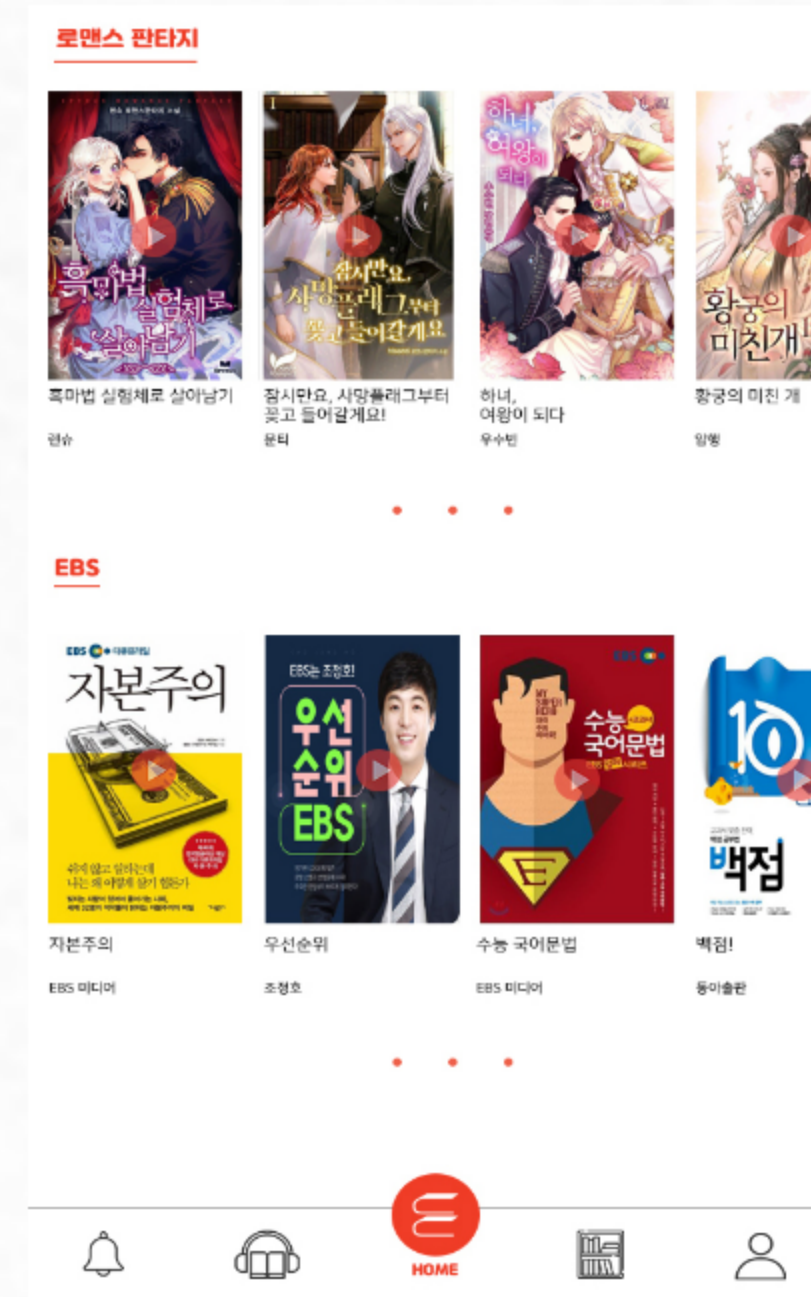
오디오북 하단
